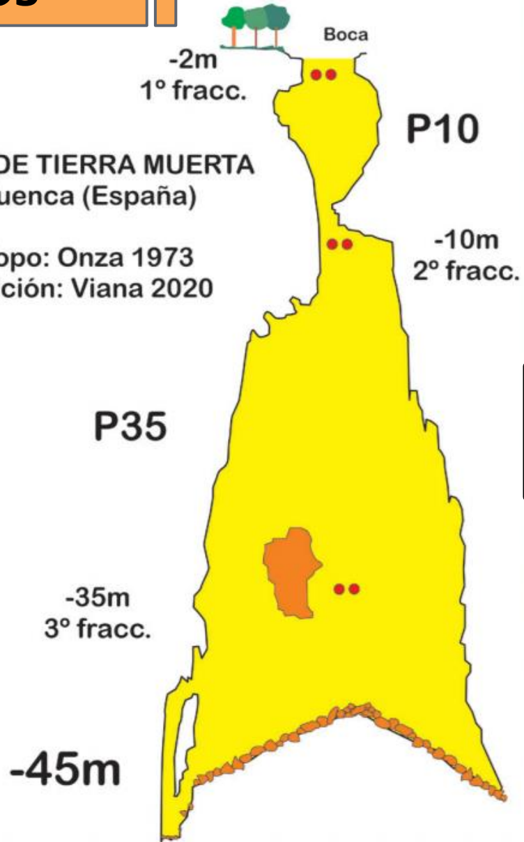
Figura 2. Sima Tierra Muerta 18/06/2019.. Valores medidos de cada una de las variables, desde la boca hasta la base. Capas de estratificación formadas según las concentraciones O 2 /CO 2 y profundidad donde se midió.
