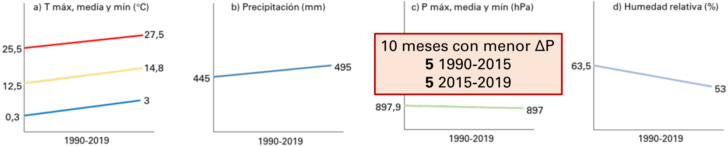
Figura 12. Gráficas periodo 1990-2019 (AEMet). Líneas de tendencia de los parámetros meteorológicos estudiados.
