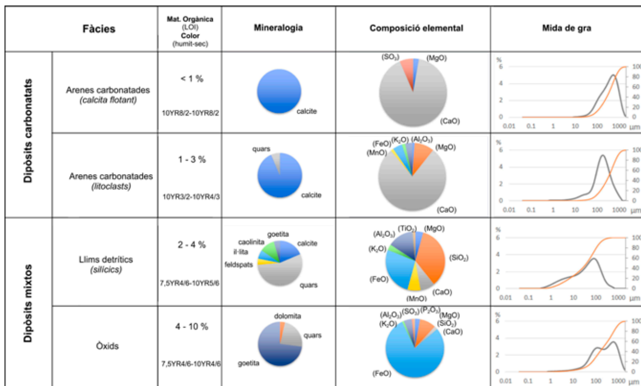
Figura 6: Característiques generals de les fàcies sedimentàries presents a la cavitat. Figure 6: General characteristics of the sedimentary facies present in the cavity.
