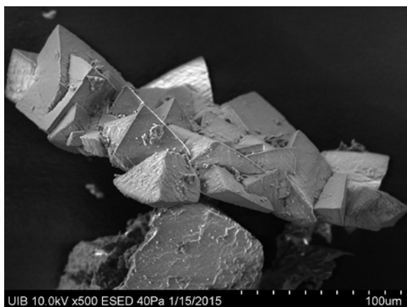
Figura 7: Imatge de microscòpia electrònica (SEM) d'un agregat de calcita flotant.
