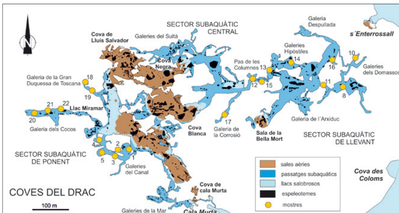
Figura 2: Mapa planimètric de les Coves del Drac amb la localització de les diferents mostres de sediment analitzades (Base topogràfica SEB –Societat Espeleològica Balear).
