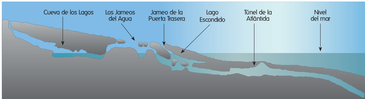
Figura 7. Mapa del perfil de las secciones anquialinas del Tubo Volcánico de La Corona. Hacia la izquierda del plano, la cueva continúa con las galerías de la Cueva de los Lagos, aunque el paso está bloqueado por un colapso. A la derecha se representa el final conocido de la cavidad, a 64 m de profundidad.
