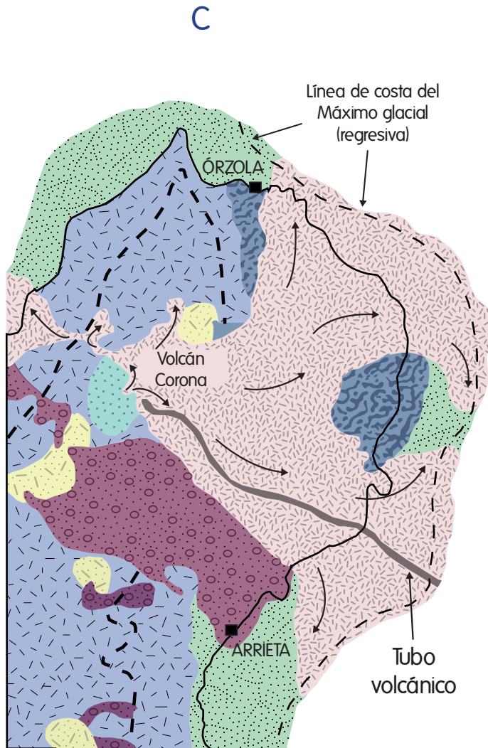
Malpaís de La Corona hace 20 Ka, durante el último máximo glacial (nivel del mar 120 m más bajo)
