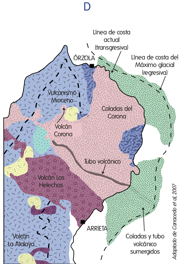
Malpaís de La Corona hoy
